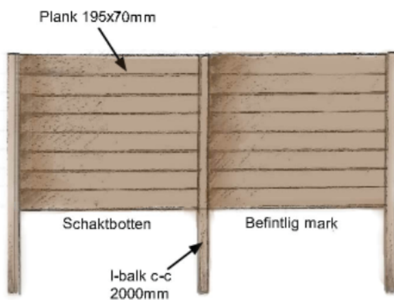
Sektioner av exempel för konstruktion av vitaliseringsdike
